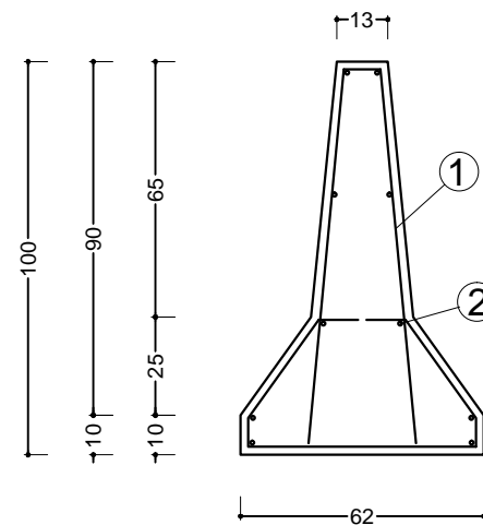
SEZIONE
