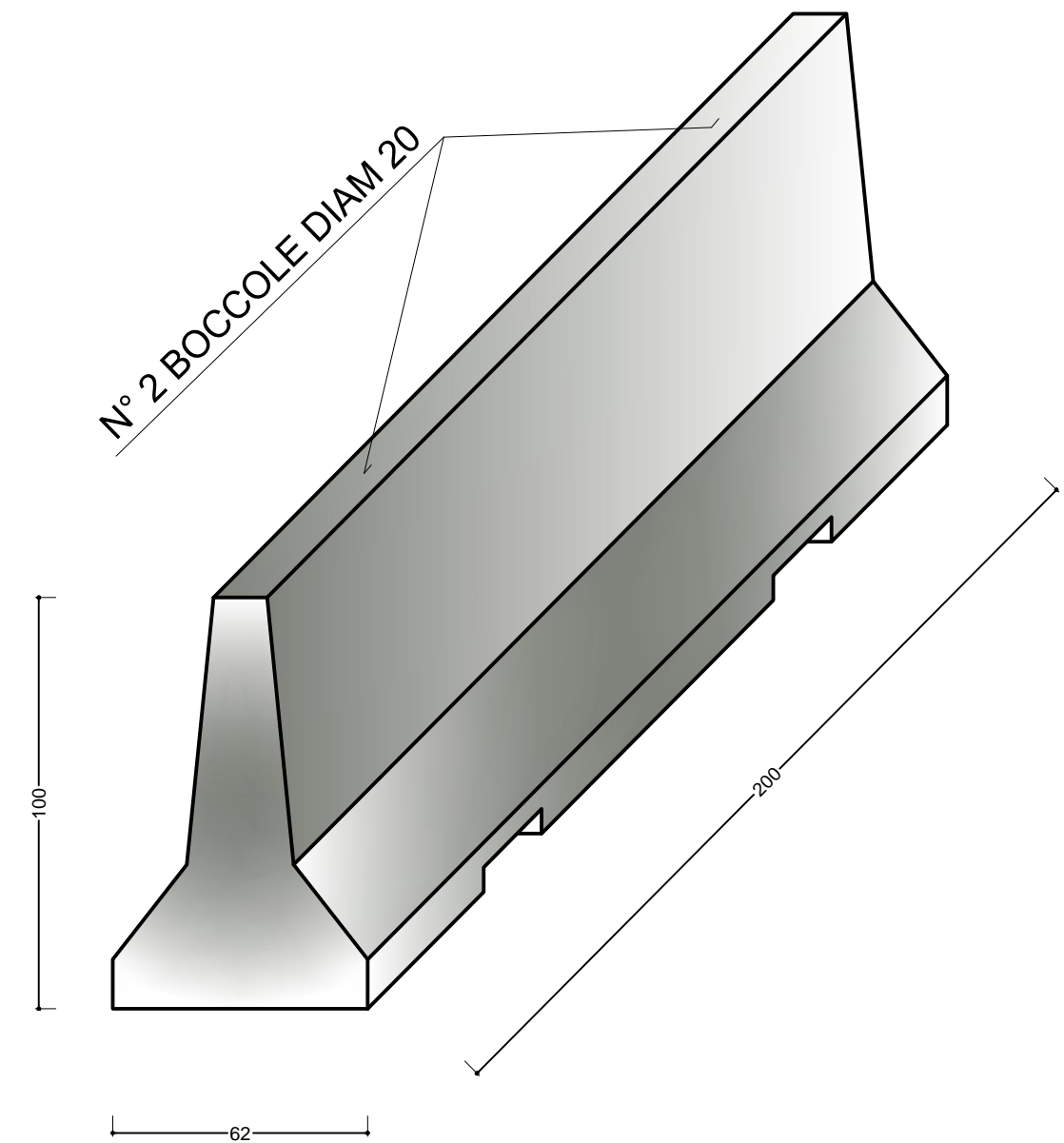
VISTA ASSONOMETRICA
